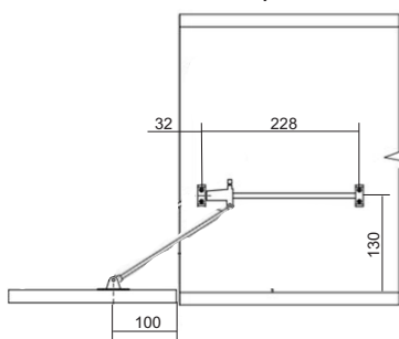
схема крепления барного кранштейна
