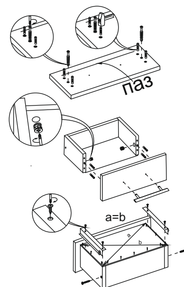
Порядок сборки выдвижного ящика
