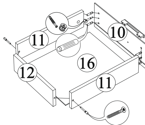
Монтаж эксцентриковой стяжки
