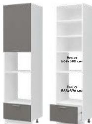
ШПМД 600 (Ф115) ШхВг 600x2130x560 мм
