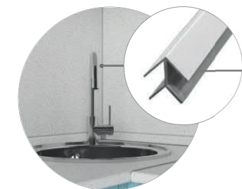
Соединитель панелей для панелей толщиной 4 мм (торцевой, угловой, щелевой)
