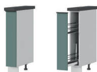
КШН 150: 150X816X495мм
