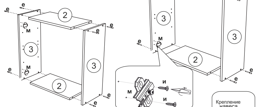
Схема крепления соед.элемента
