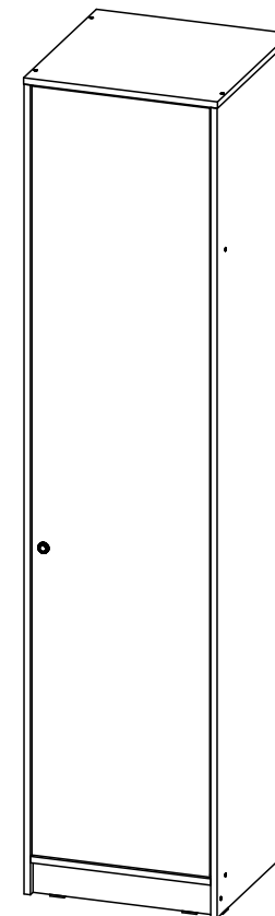
«Киви» ШК-01 Шкаф-пенал ↔485 ↑2038 ↗503 «Kivi» ShK-01 Wardrobe-case
