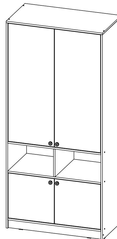
«Киви» ШК-02 Шкаф 2ств ↔934 ↑2038 ↗503 «Kivi» ShK-02 Wardrobe 2stv
