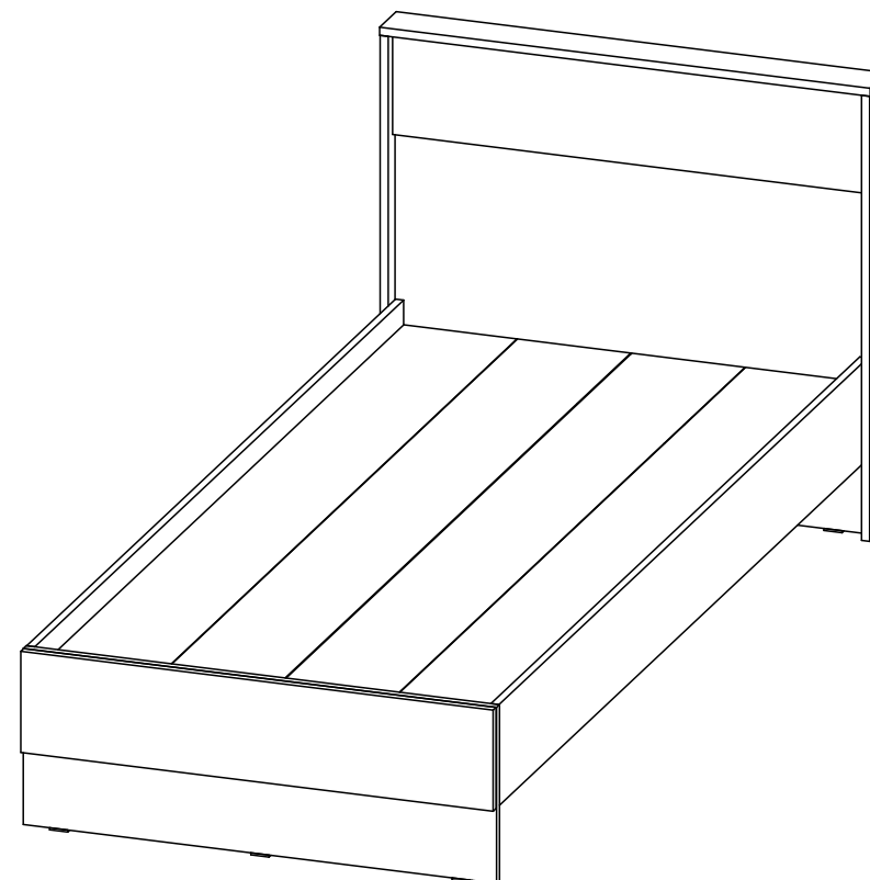
«Ирис» КР-01 Кровать 0,9х2,0 ↔ 970 ↑ 900 ↗ 2090 «Iris» Kr01 Bed 0,9x2,0
