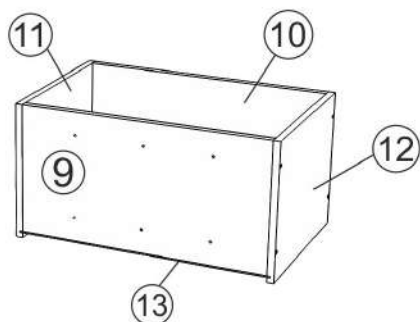
Рис.4 Ящик выдвижной.
