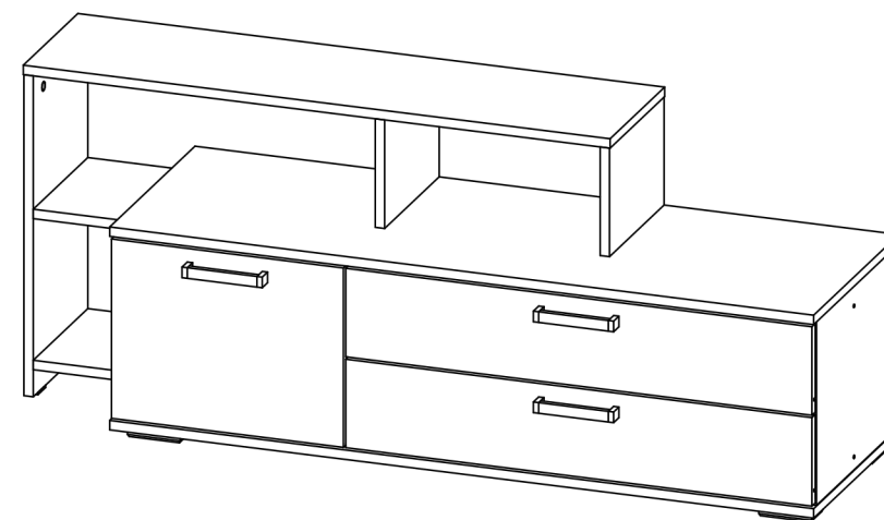
«Санса» TB 01 Тумба под ТВ ↔ 1400 ↑ 565 ↗ 400 «Sansa» TB 01 TV cabinet
