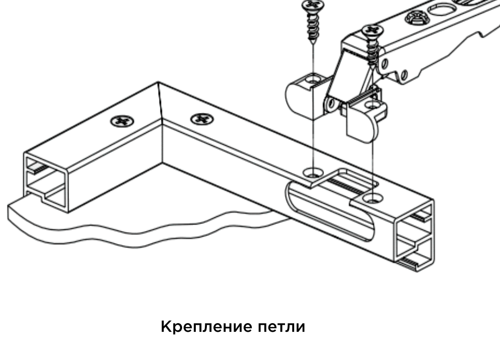
Крепление петли
