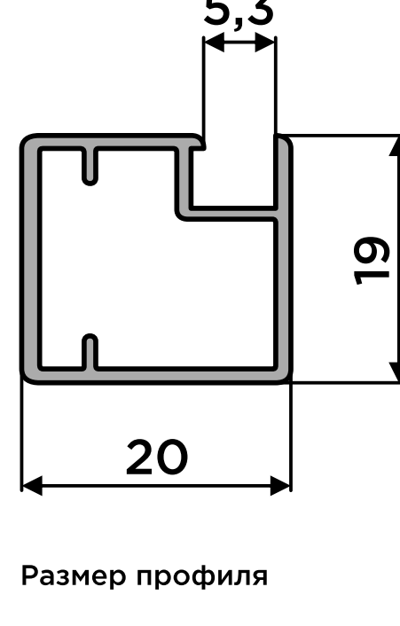
Размер профиля
