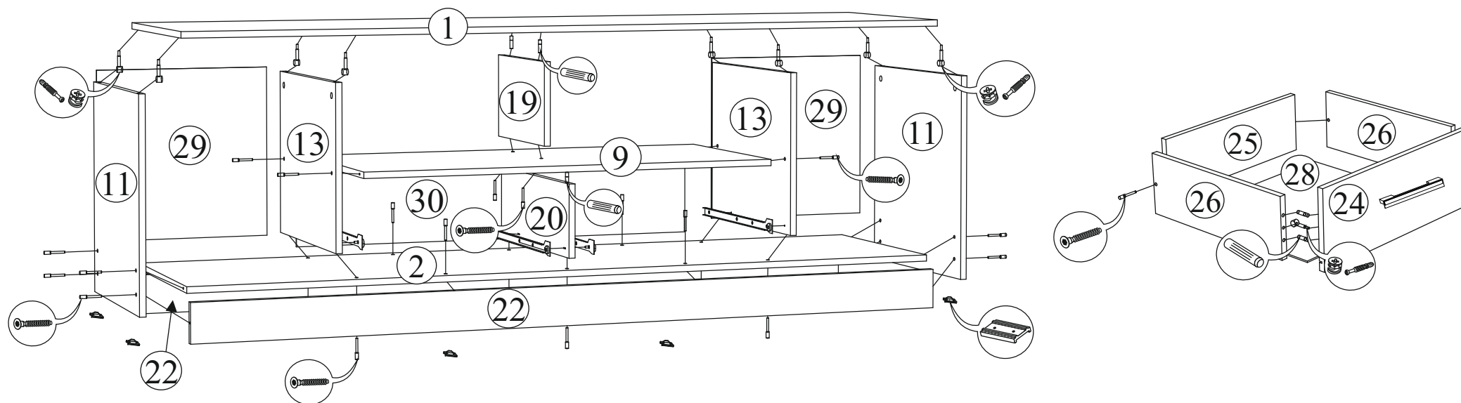
Рис. 1. Рассверловка перегородки
