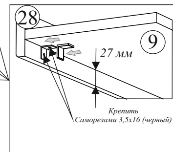
Схема крепления планок № 28.
