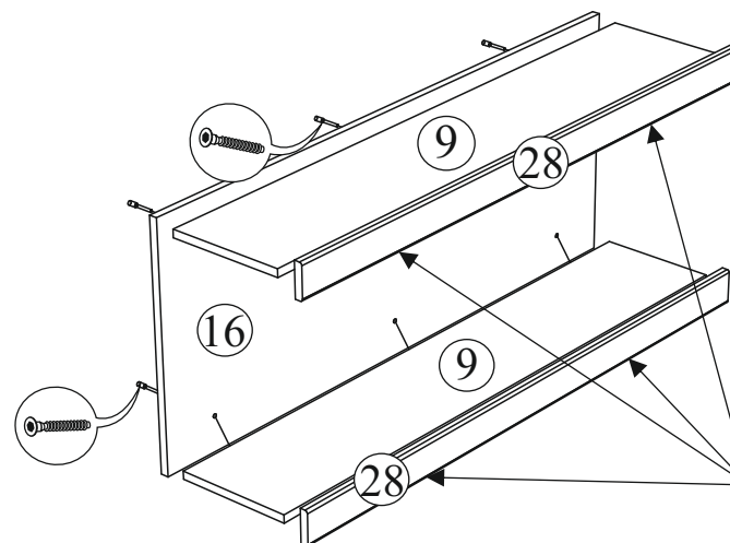
Схема крепления планок № 28.
