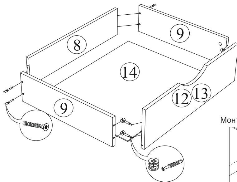
Схема сборки ящика
