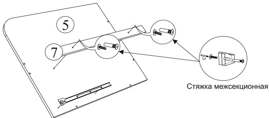
Схема сборки ящика
